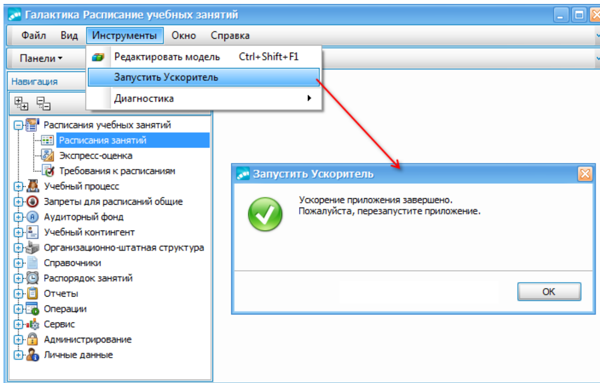
Рис. 30. Запуск ускорителя
