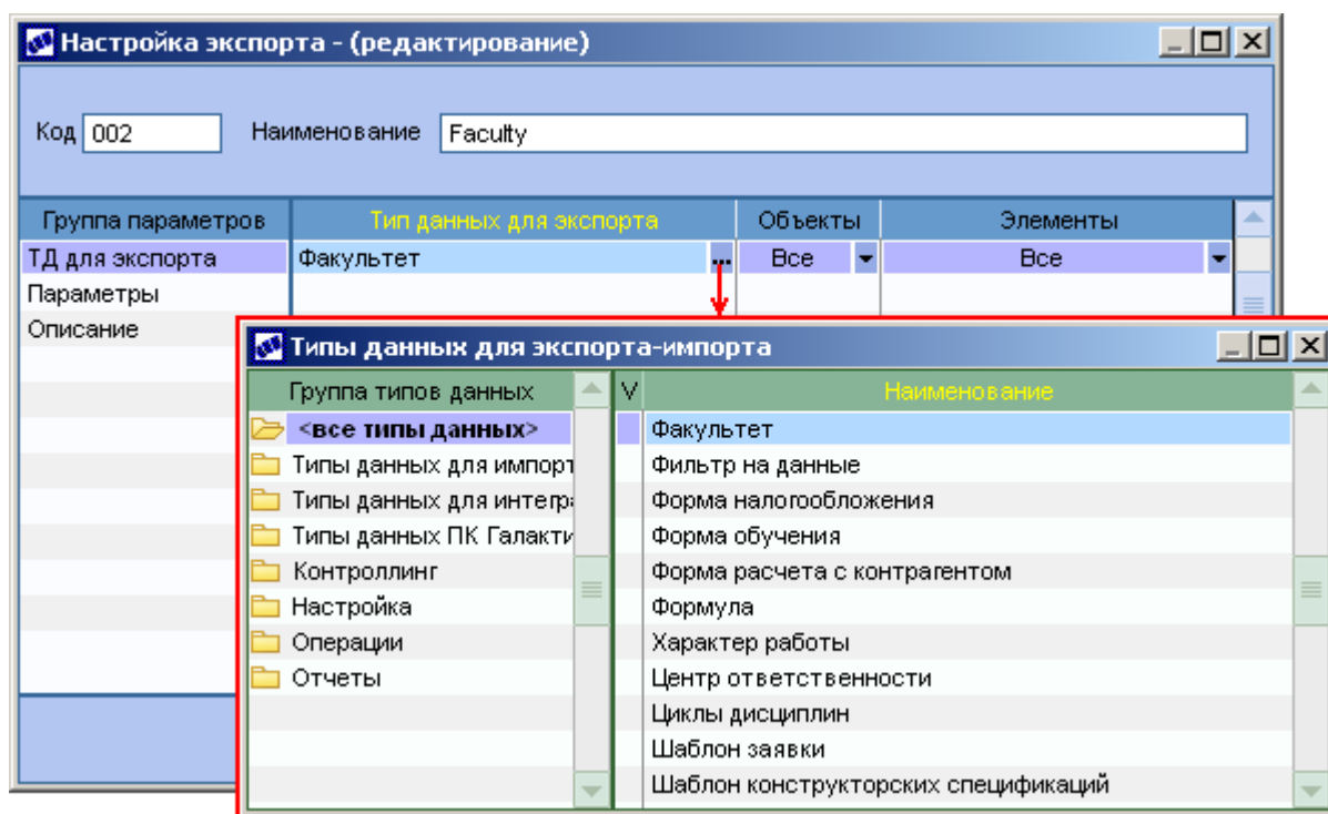
Рис. 37. Настройка экспорта
