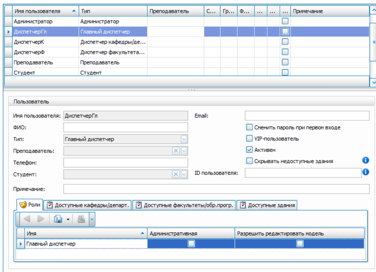
Рис. 27. Пользователи системы
