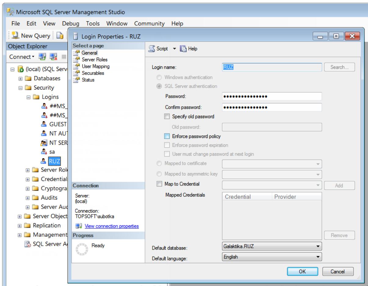
Рис. 20. Создание пользователя в MS SQL Server
