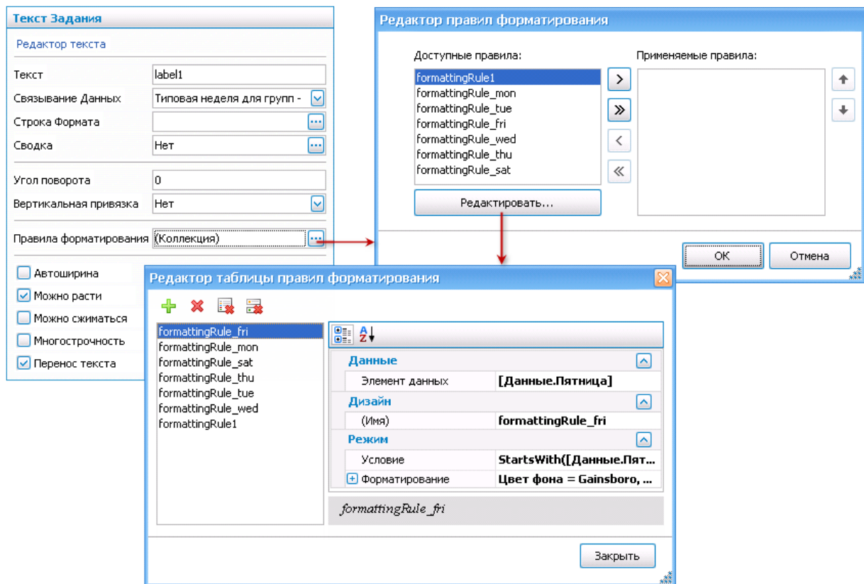
Рис. 46. Правила форматирования
