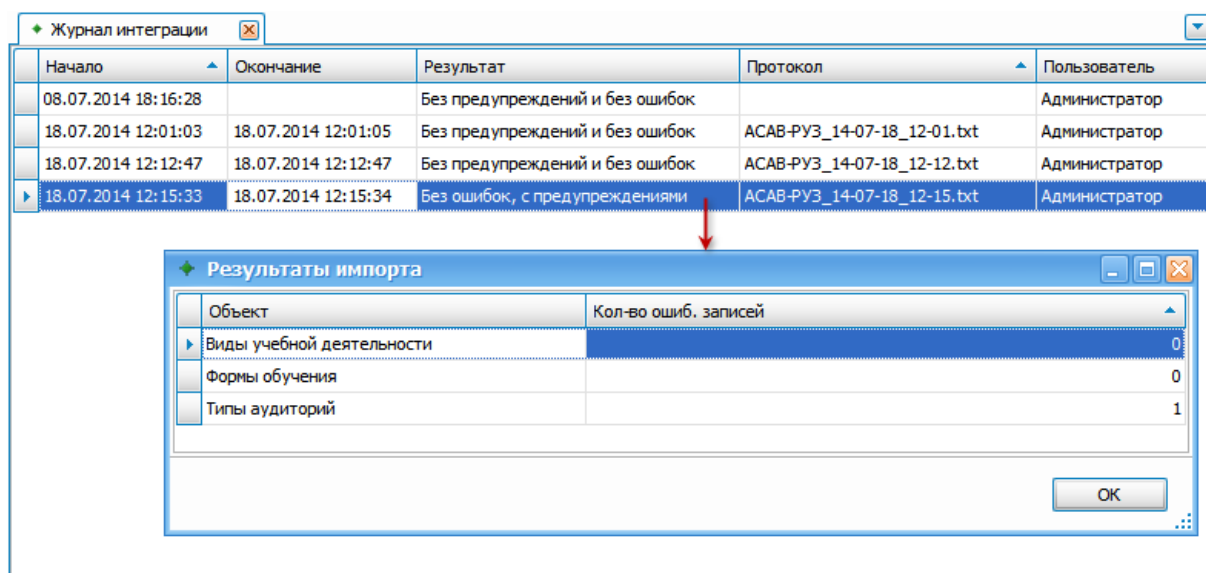
Рис. 39. Журнал интеграции
