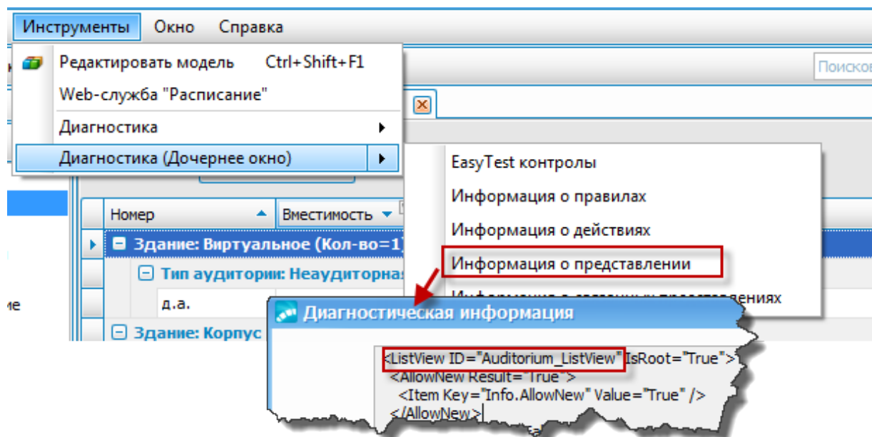
Рис. 51. Диагностическая информация
