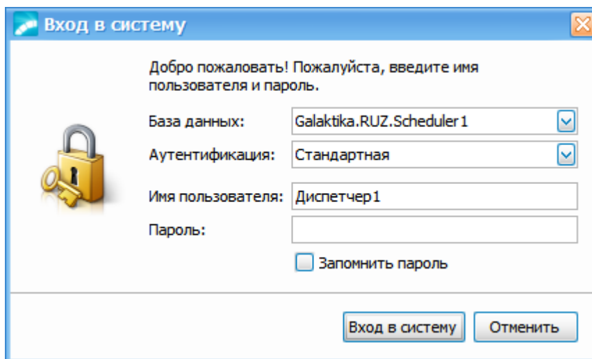
Рис. 23. Авторизация
