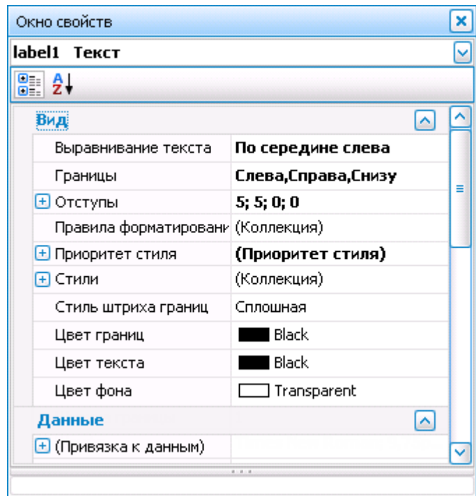
Рис. 45. Окно свойств
