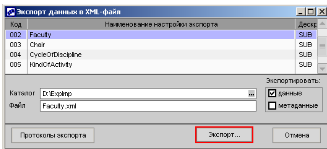
Рис. 38. Экспорт
