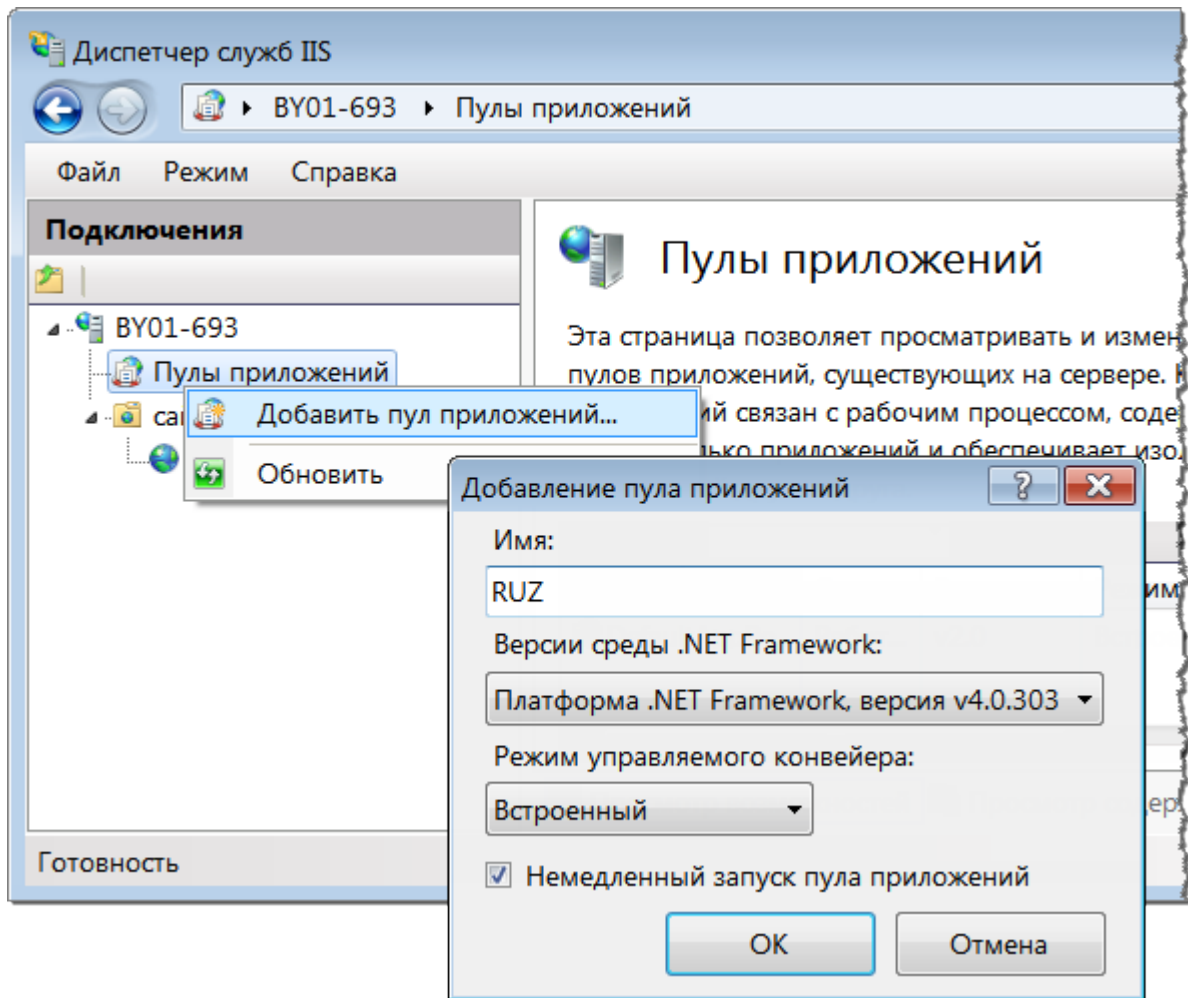
Рис. 12. Создание пула
