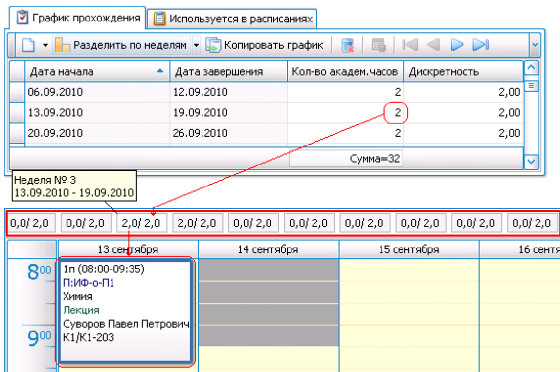
Рис. 46. График прохождения нагрузки
