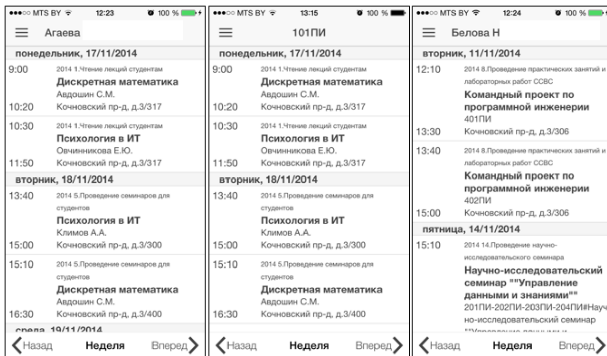
Рис. 81. Просмотр расписания
