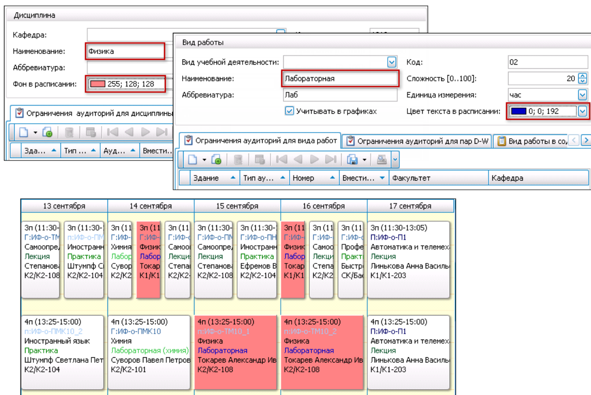
Рис. 50. Цветовое выделение информации
