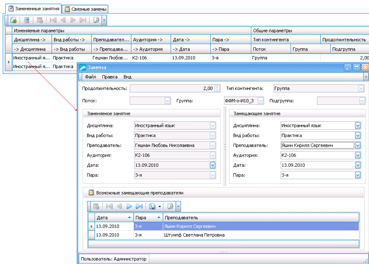
Рис. 64. Замена
