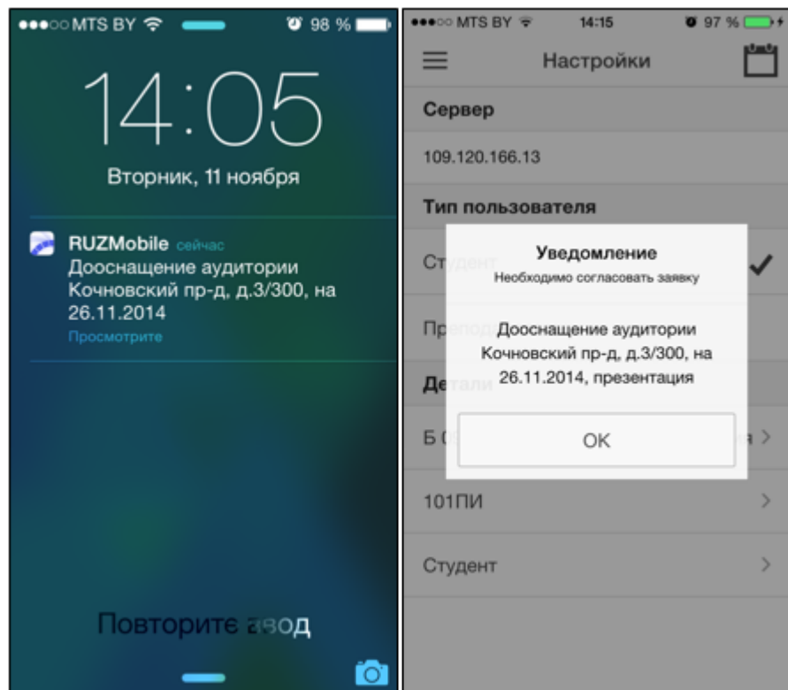
Рис. 84. Получение уведомления
