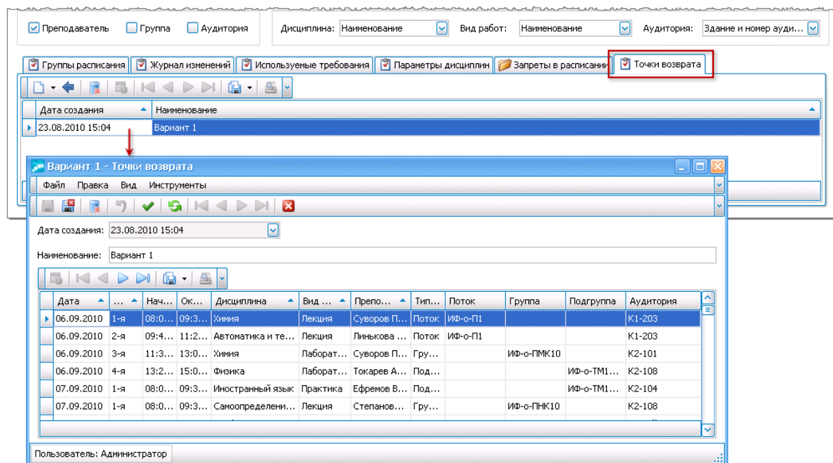
Рис. 66. Точки возврата
