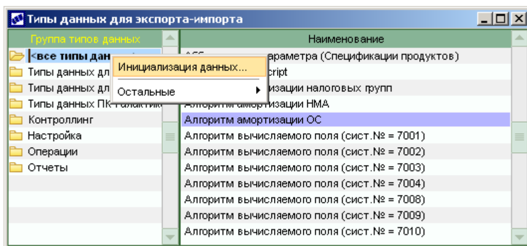
Рис. 40. Инициализация данных
