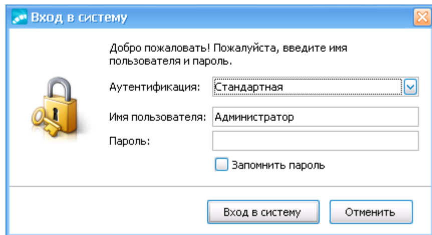
Рис. 13. Стандартная аутентификация
